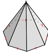
pirámide heptagonal
