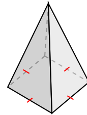
pirámide cuadrada
